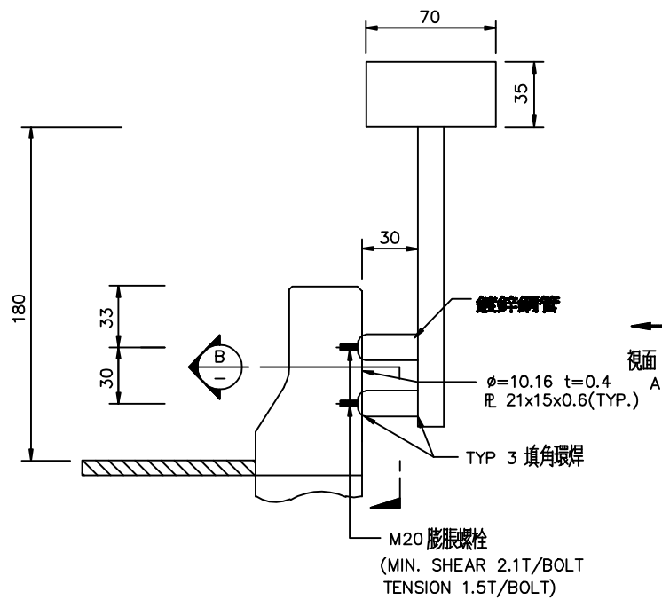
外側附掛式公里里程牌 (B 型)
